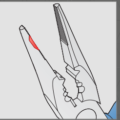
Kemény vezetékek felcsavarásához és gyűrűk hajlításához 3.5 mm átmérőig. Gyűrűk jobb és bal irányba is hajlíthatók, mivel a fogók mindkét oldalon rendelkezik a megfelelő fogazással.
