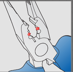
Szigetelés eltávolítása 2.2 - 3.0 mm átmérőjű vezetékeknél.
