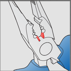
Vezetékek vágása 2.2 mm - 4.0 mm átmérők között.
