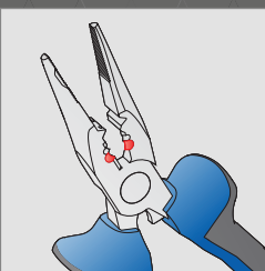
Szigetelés eltávolítása 3.5 - 4.0 mm átmérőjű vezetékknél.
