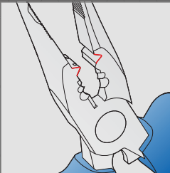
A fogó használható szigetelt kábelsaruk préseléséhez.
